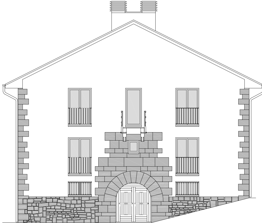
ALZADO NORTE
